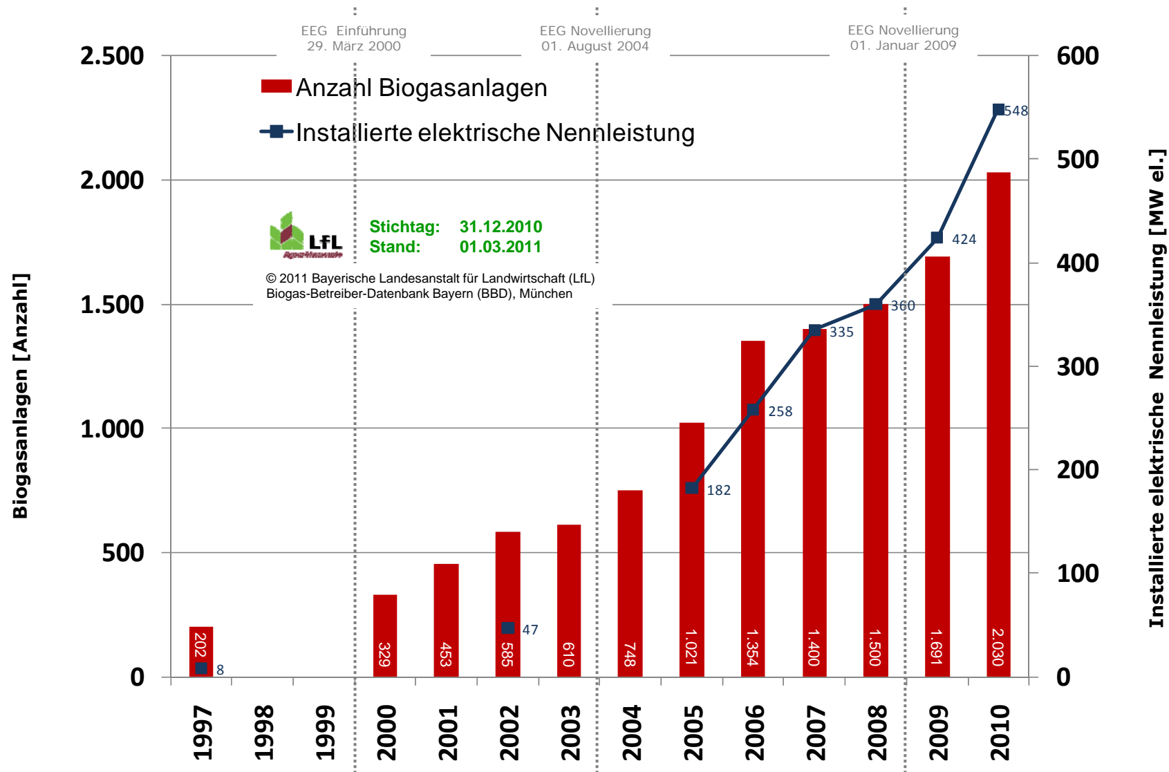
Abbildung 1: Zeitreihe zur Anzahl der Biogasanlagen und zur installierten elektrischen Nennleistung [MW el.] in Bayern zum 31.12.2010
