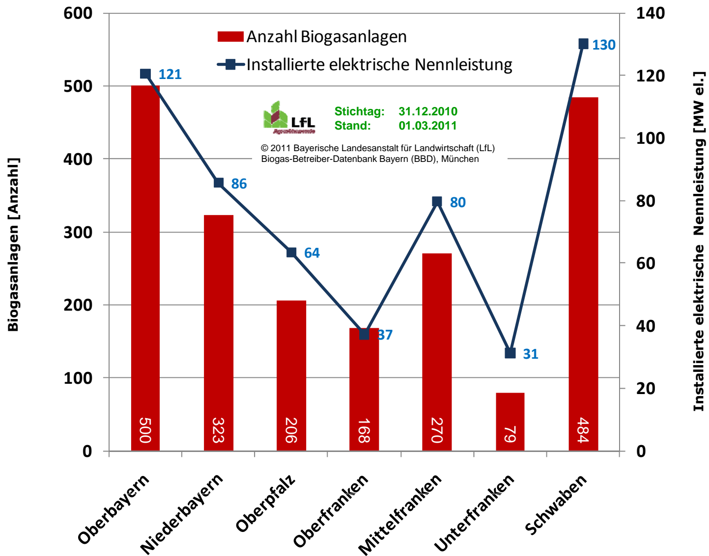
Abbildung 2: Anzahl der Biogasanlagen und installierte elektrische Nennleistung [MW el.] nach Regierungsbezirke in Bayern zum 31.12.2010
